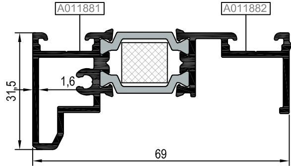
ATP64A28 (KATLANIR İÇİN)
